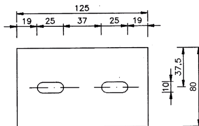
Abb. 2: Rückwand SchlüsselDepot K3
