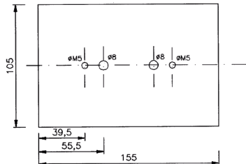
Abb. 3: Grundplatte (optional)
